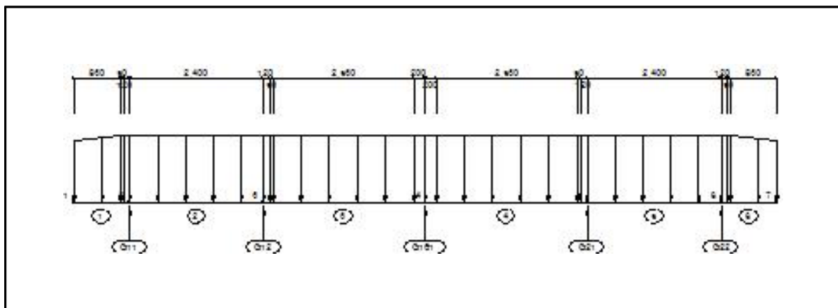
【그림 2.3.9】 바닥판 자중 횡방향 하중분배
