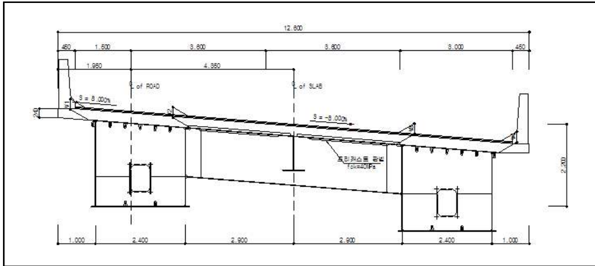
【그림 2.3.8】 해석단면
