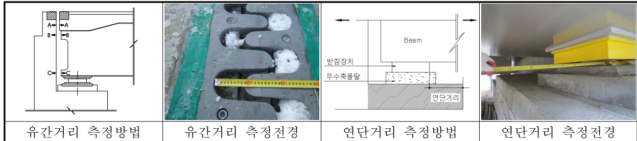
【그림 2.3.6】 부재별 기능상태 측정방법 및 전경
