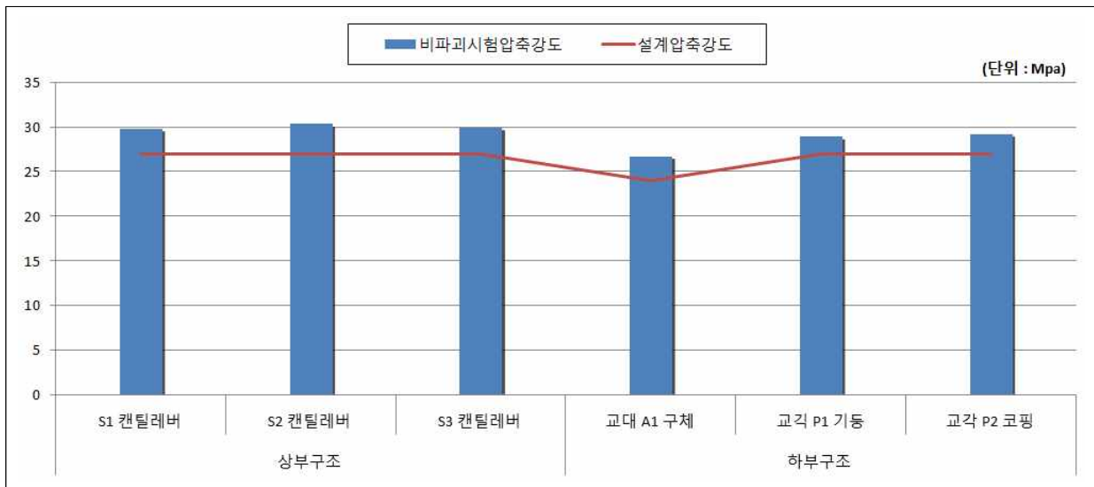
【그림 2.3.7】 콘크리트 강도시험 결과 그래프
